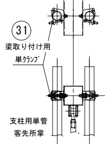
① 梁、支柱用単管 取り付け要領図
