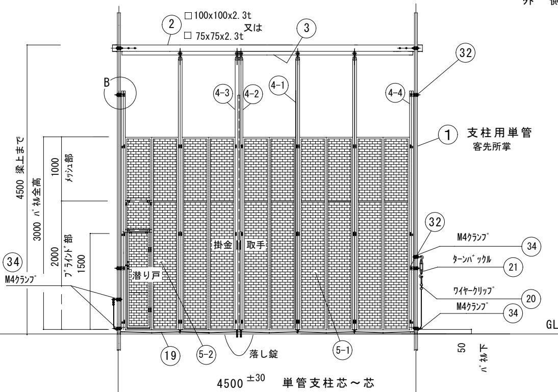
正面図
