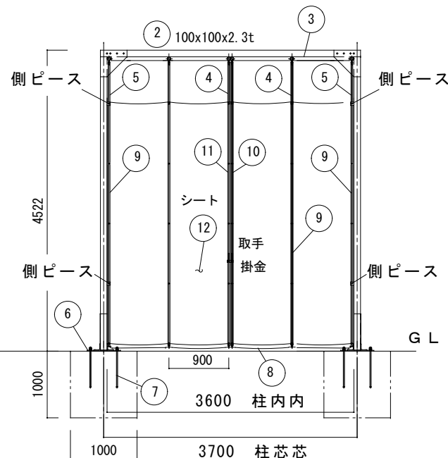
正 面 图
